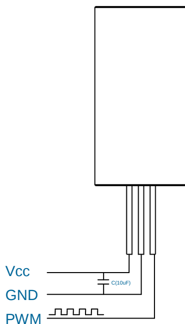
PWM mode
